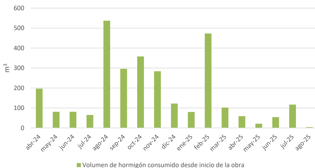
Figura 3-5 Consumo de hormigón desde el inicio de la obra.
