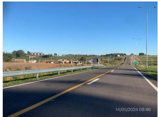
Foto 12.2-4, Ruta 27, obras terminadas. Carpeta de rodadura en mezcla asfáltica ejecutada.
